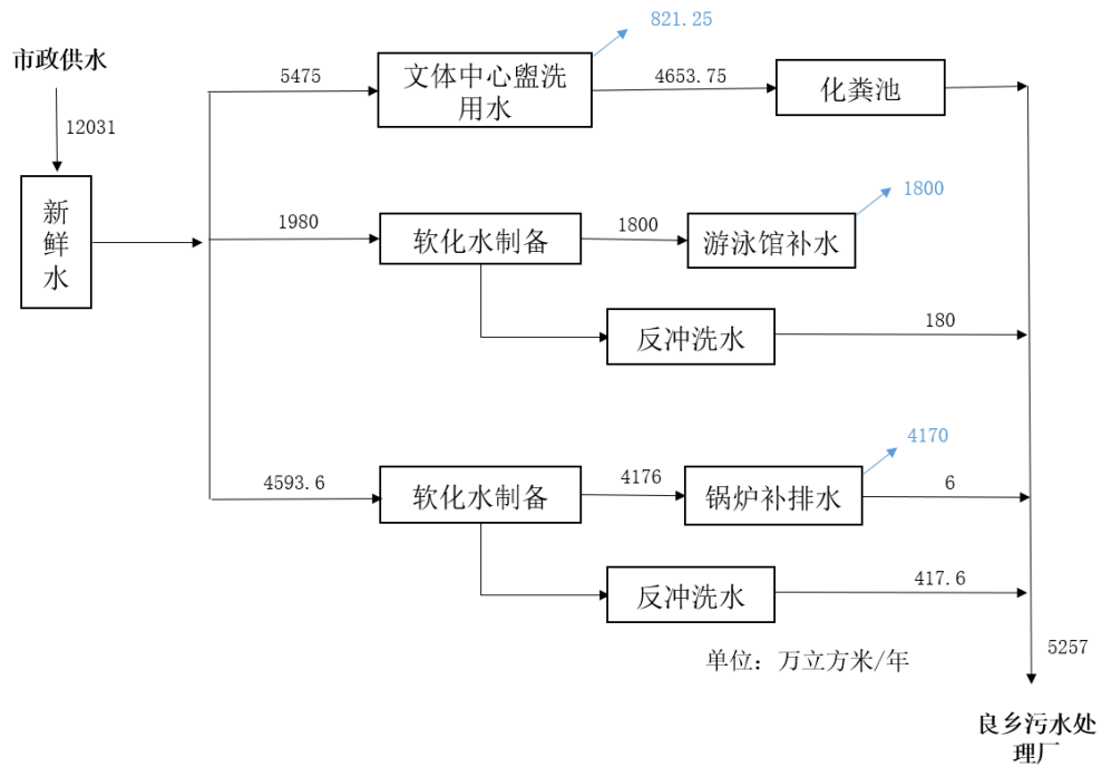
图3-11 水平衡图
